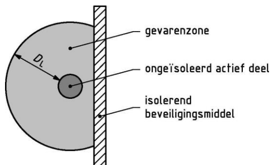
Figuur 2 – Gevarezone bij gebruik van een isolerend beveiligingsmiddel.
